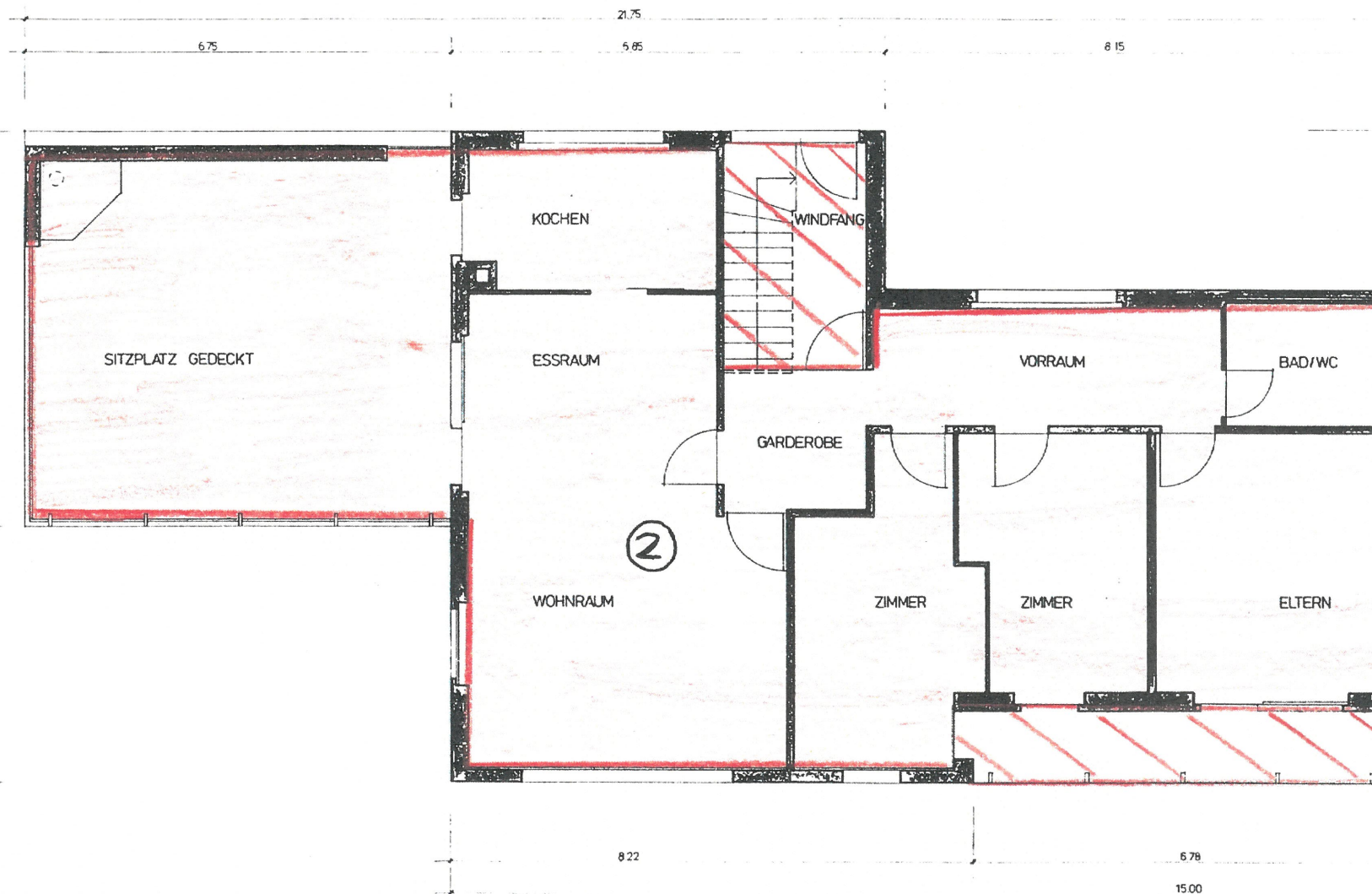
ERDGESCHOSS
